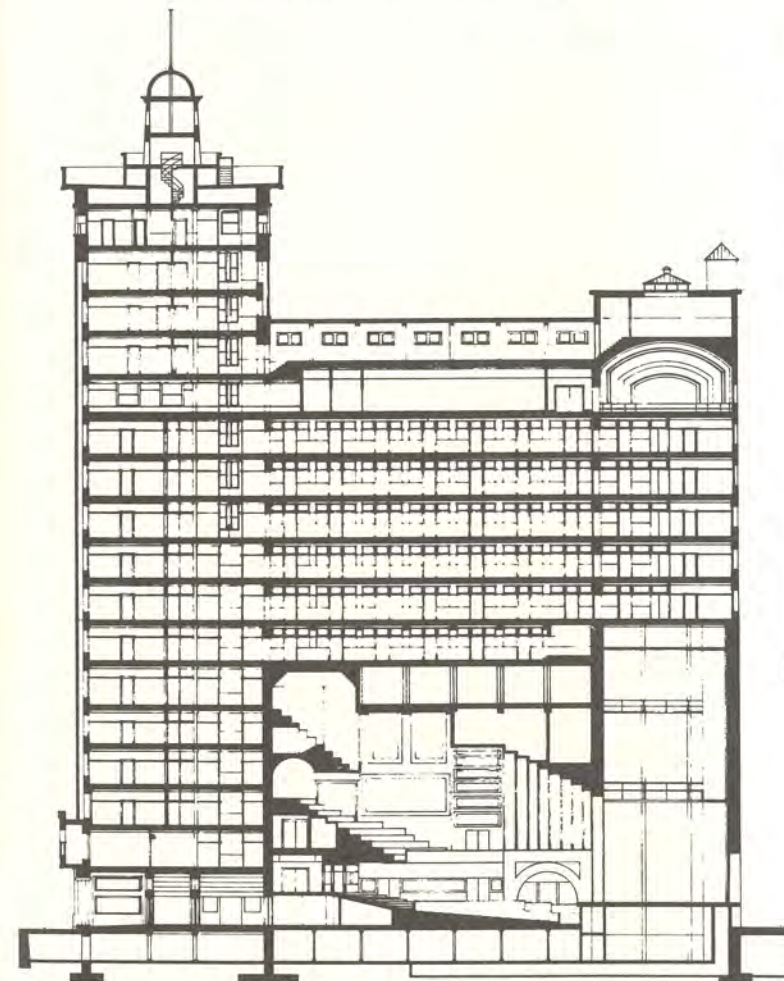
LONGITUDINAL SECTION
